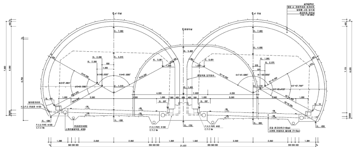
&lt;횡단면도&gt;
